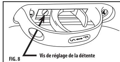
FIG. 8 Vis de réglage de la détente
